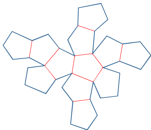
十二面体
